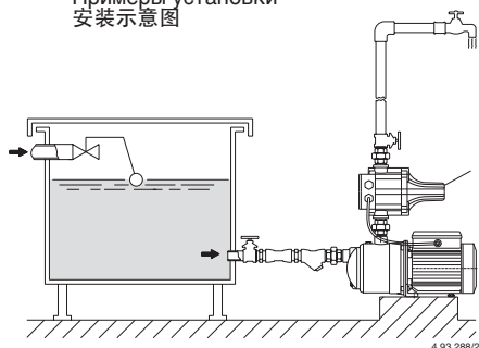
Fig. 1 Funzionamento sotto battente Positive suction head operation Zulaufbetrieb
