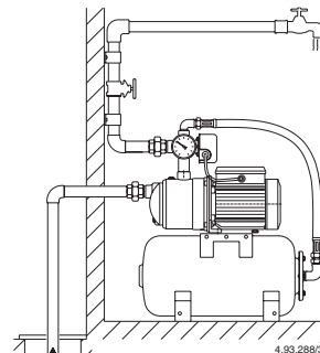
Fig. 2 Funzionamento in aspirazione Suction lift operation Saugbetrieb
