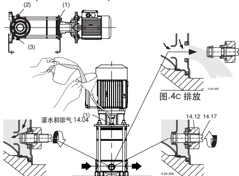
图.4a 灌水： 内部通道打开
