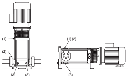
ΦΣχ. 46. (1) Γέμισμα και εξαέρωση (2) πρόσληψη εξαερισμού (3) Αποστράγγιση
