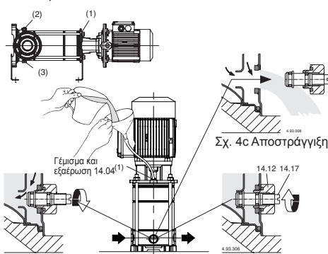
Σχ. 4a Γέμισμα:
