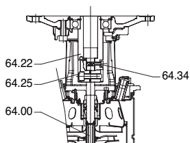
Abb. 6a Stehender Läufer, Welle nicht blockiert in Kupplung (*) Stift für Wellenanheben.
