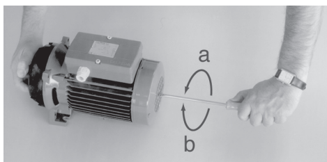
图5 拆卸(a)和回装(b)叶轮
