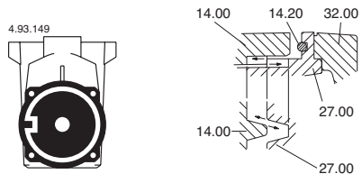
Abb. 6 Montagenut für Zusammenbau Pumpengehäuse (14.00) - Diffusordeckel (27.00)
