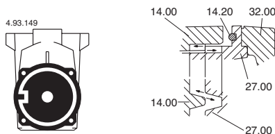
Fig. 6 Vervangen pomphuis (14.00) - diffuserdeksel (27.00)
